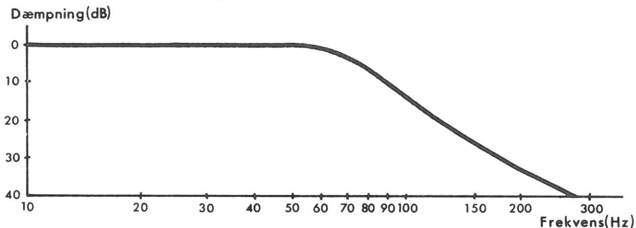
Fig. 6 LAVPASFILTER.
